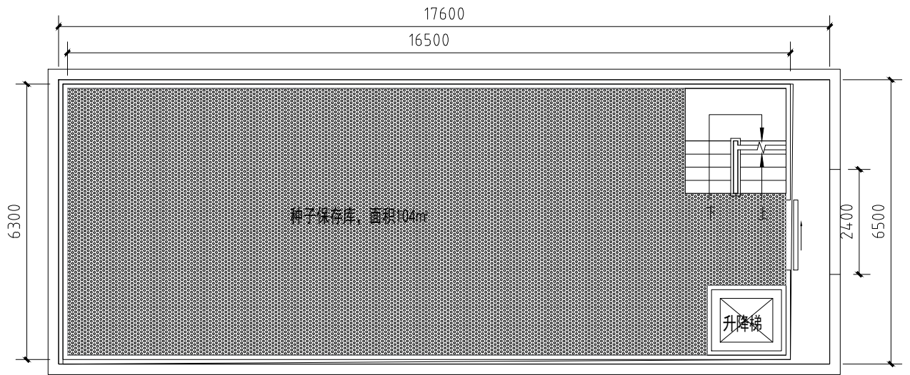
种子保存库, 吊顶4500, 层高5900,
